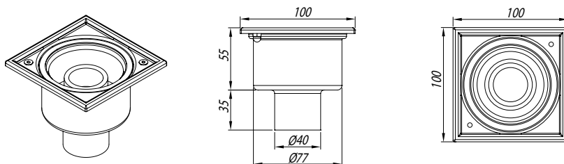
Трап горизонтальные
