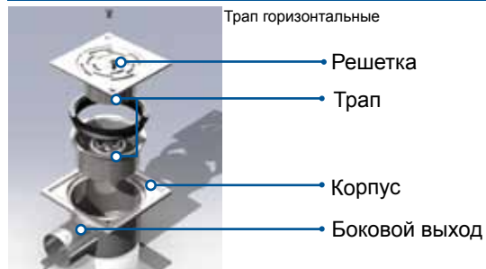
Трап горизонтальные
