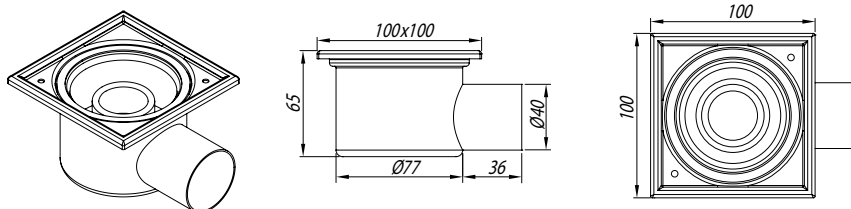
Трап горизонтальные
